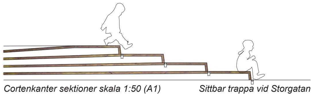
Cortenkanter sektioner skala 1:50 (A1)
